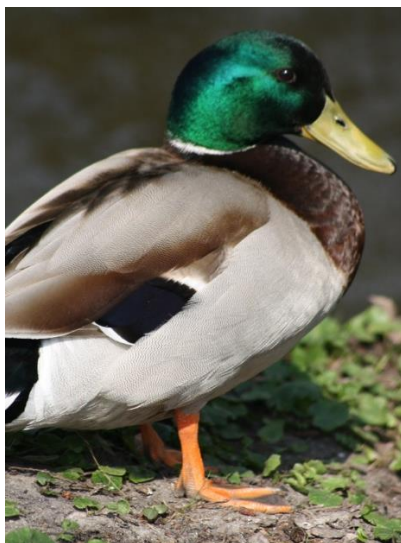
Gräsand ( Anas platyrhynchos )
